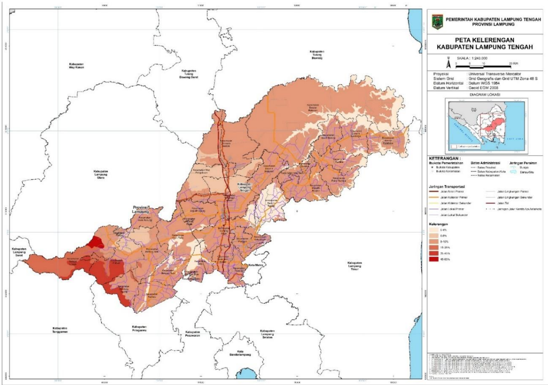
Gambar 2.3 Peta Kelerengan Kabupaten Lampung Tengah
