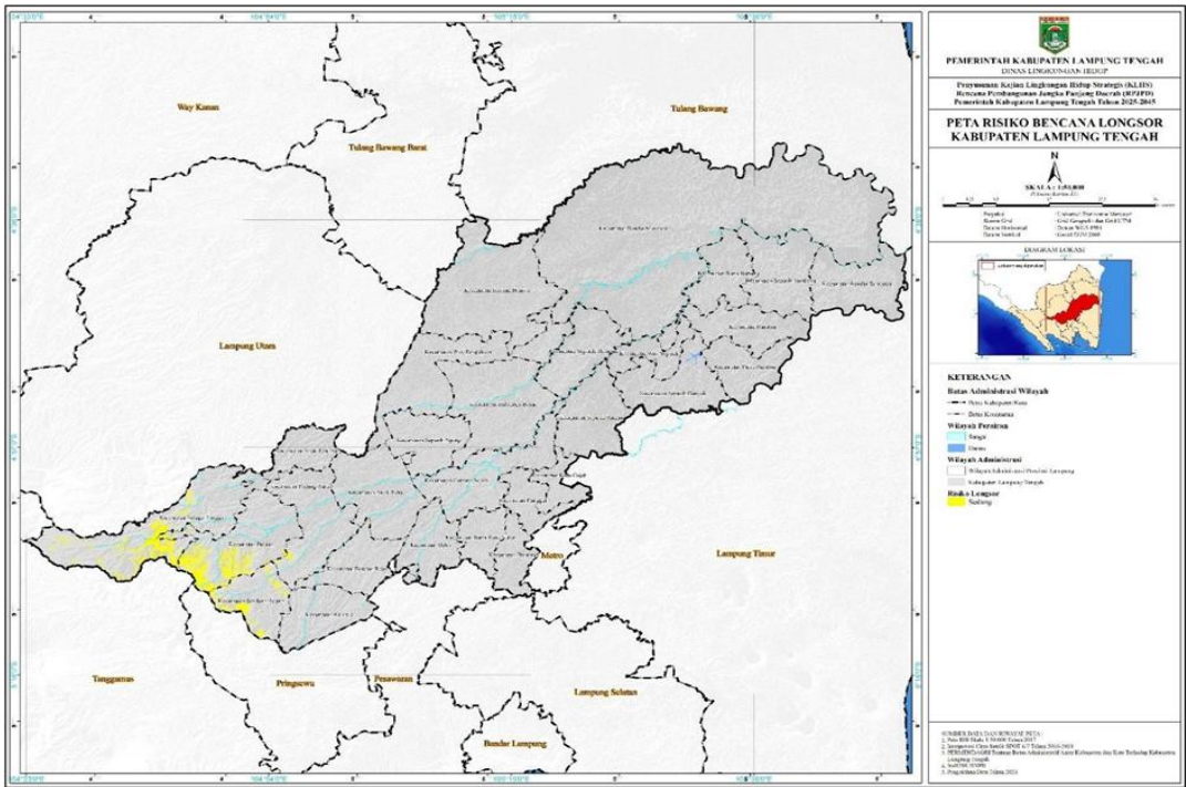
Gambar 2.10 Peta Risiko Bencana Longsor
